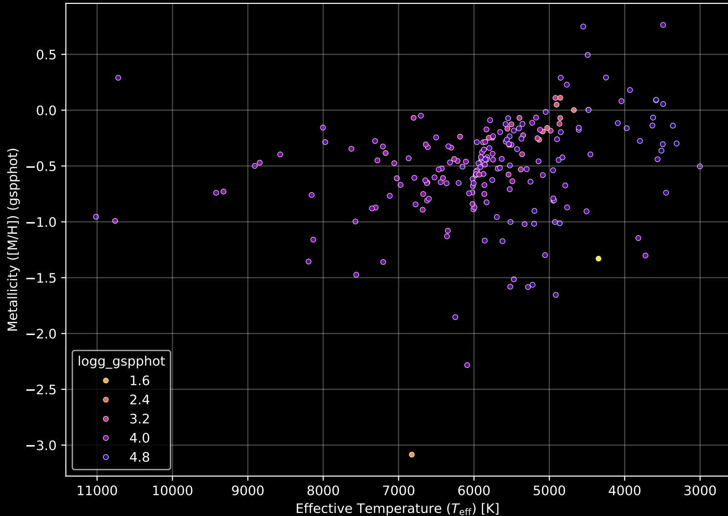
APOGEE DR17 Field: [K2_C13_176-17_btx] Stellar Population Parameters (n= 206)
